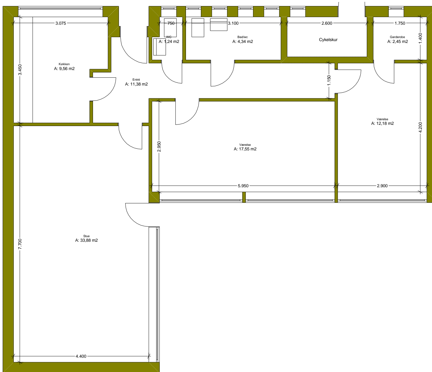
Stueplan
