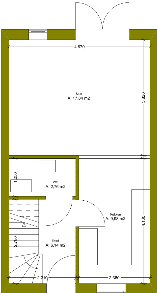
Stueplan
