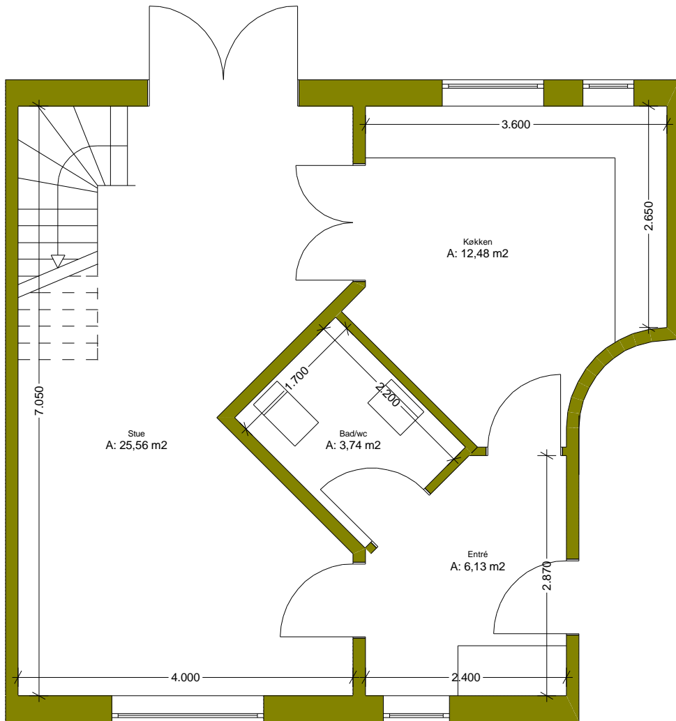
1. salsplan
